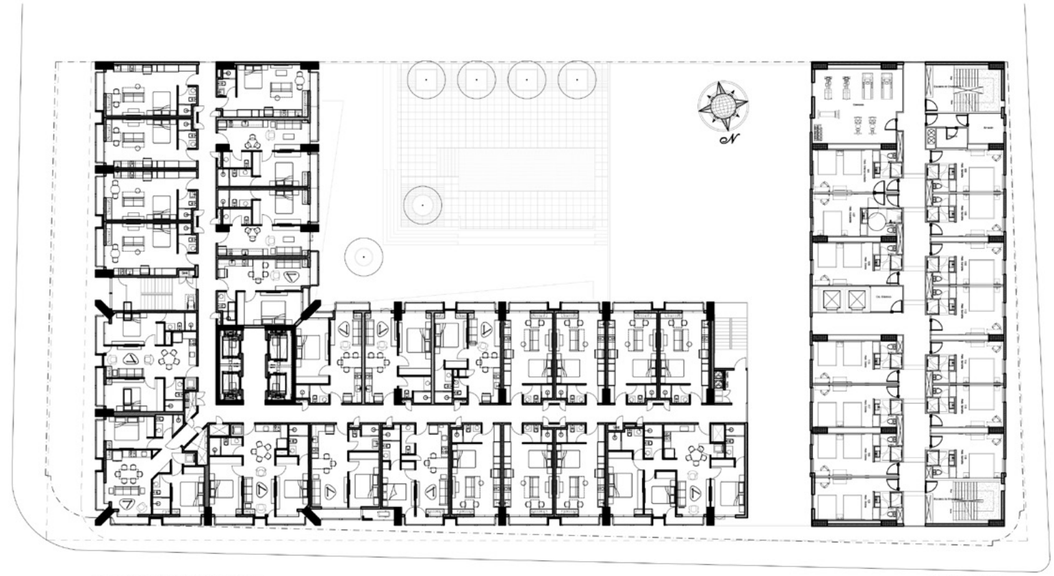
PLANTA TIPO DEPARTAMENTOS
